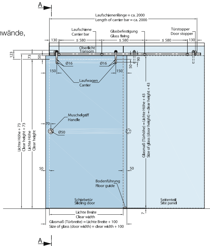
Glas-Schiebetüre mit Oberlicht und Seitenteil
