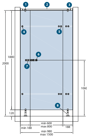
Haltewinkel für Kabinenzwischenwand WC-Trennwand
